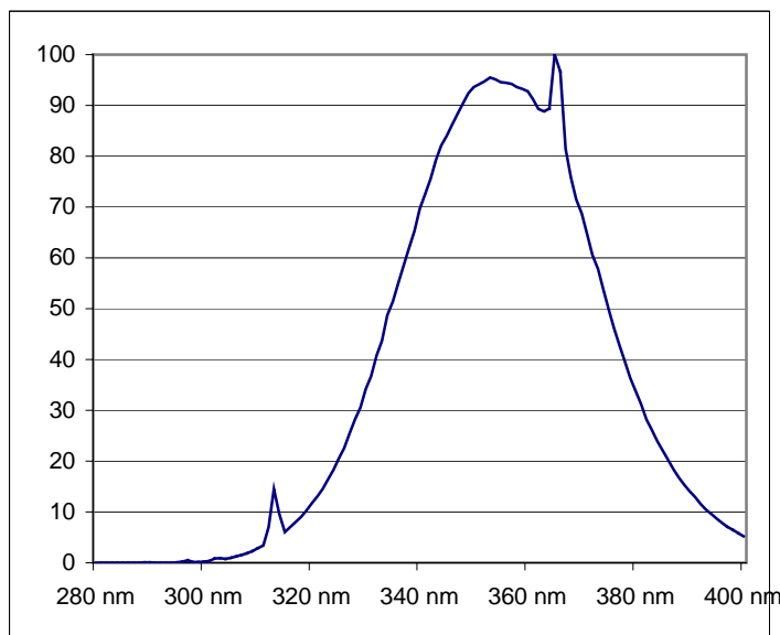
Relativer spektraler Strahlenfluss (280 – 400) nm Relative Spectral Radiant Flux (280 – 400) nm
